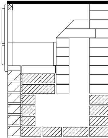
B-B
